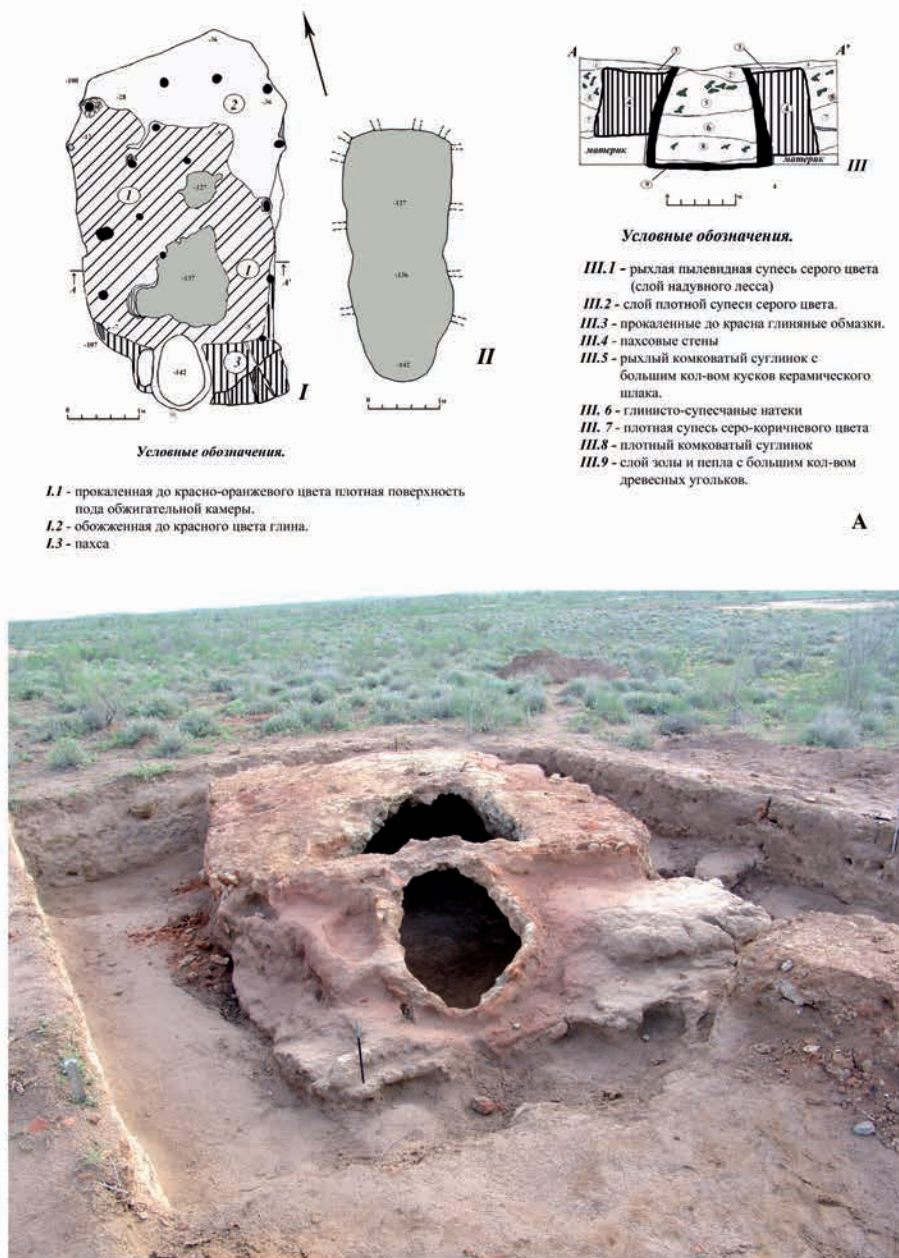
А- горн №1. План и разрез топочной камеры. Б- горн №1. Фото, вид с юга.
